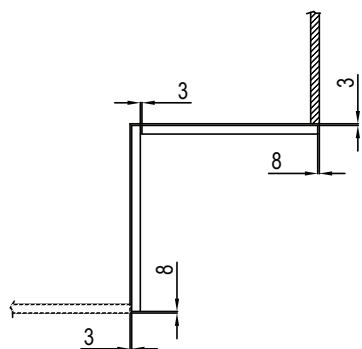
Door panel - pattern 1 Panneau de porte - modèle 1
