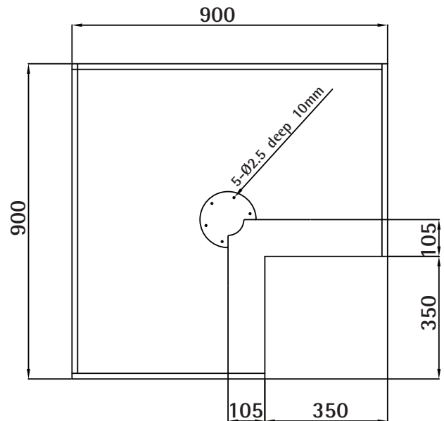
For the upper panel Pour le panneau du haut
