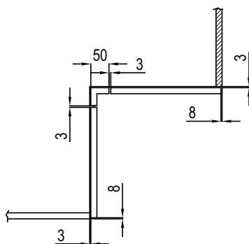
Door panel - pattern 2 Panneau de porte - modèle 2
